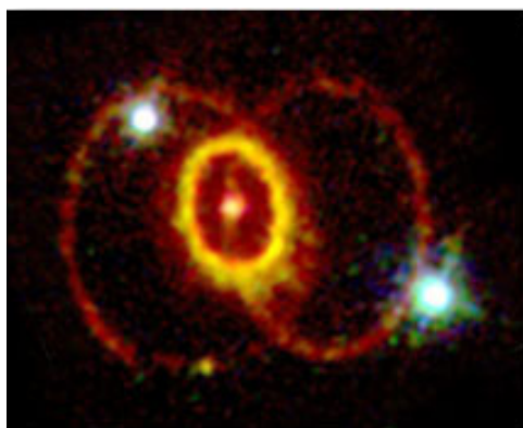
Supernova 1987A.
